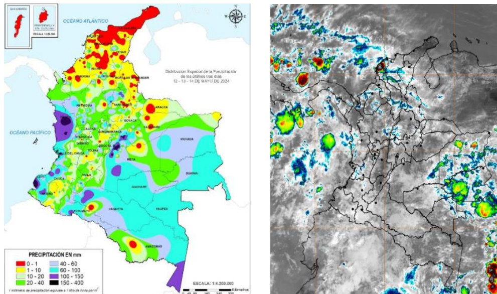
Imagen GOES East Canal Infrarrojo - Mapa de precipitación últimas 72 horas desde las 07:00 HLC del domingo 12, hasta las 07:00 HLC del miércoles, 15 de mayo de 2024. Fuente: IDEAM
