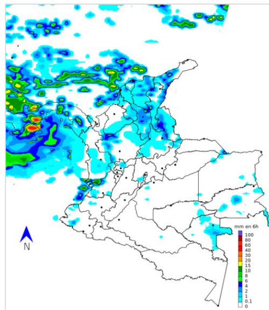
Pronóstico de precipitación acumulada en 06:00 horas a partir de:2024-08-30 07:00 HLC
